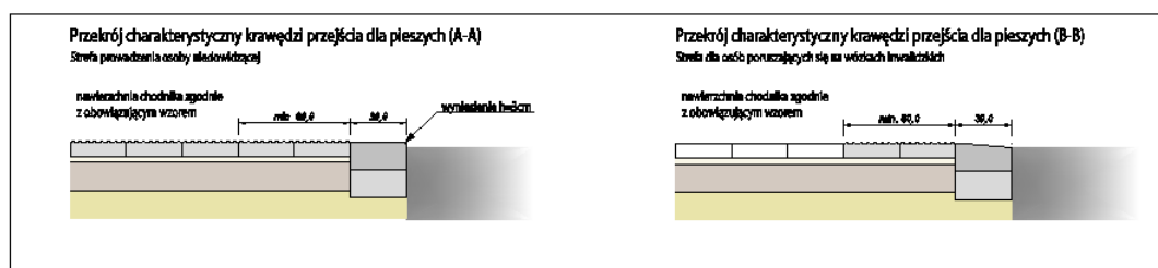
Przekroje charakterystyczne przejścia dla pieszych
